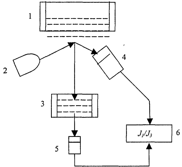
Рис. 2. Схема измерения с использованием дополнительного поглотителя: 1 - образец; 2 - источник излучения; 3 - поглотитель из анализируемого вещества; 4 - детектор излучения; 5 - детектор излучения; 6 - блок регистрации
