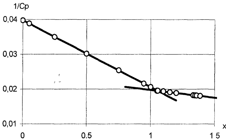
Рис. 2. Зависимость стандартной кельджи (обратной величины стандартной молярной теплоемкости) оксидов железа FeO_x от их состава, отнесенному к одному молю железа. Левая ветвь – I область т.р., правая ветвь – II область т.р.
