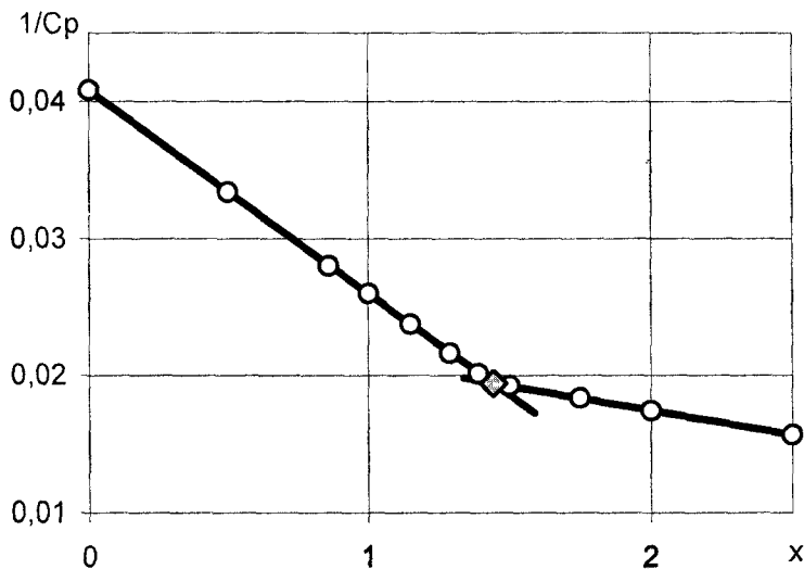
Рис.1. Зависимость стандартной келджи (обратной величины стандартной молярной теплоемкости) оксидов ванадия VO_x от их состава, отнесенной к одному молю ванадия. Левая ветвь – I область т.р., правая ветвь – II область т.р.
