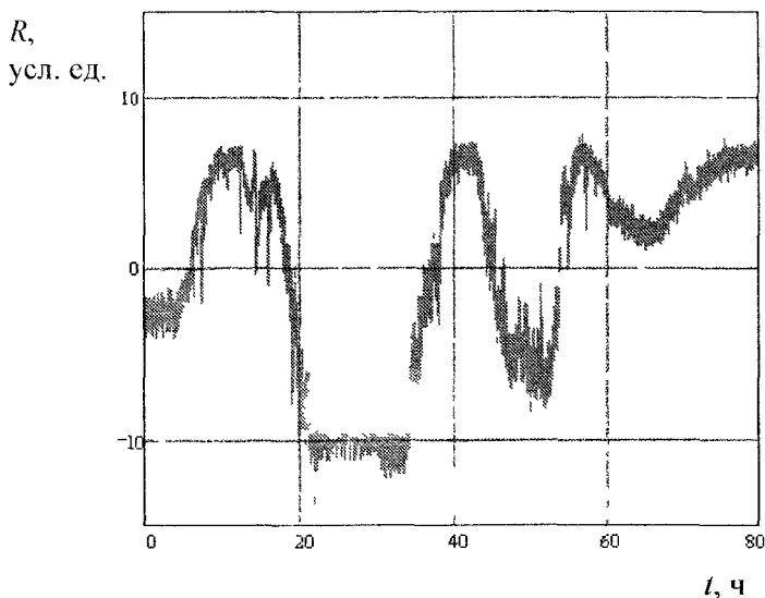
Рис. 1. Изменение сопротивления детектора во времени
