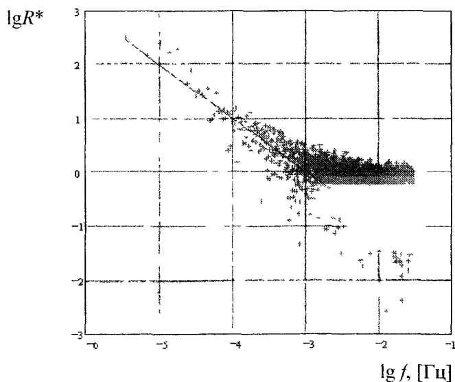
Рис. 2. Спектр флуктуаций сопротивления. Сплошная линия – ожидаемый спектр фликкер-шума ( 1/f )
